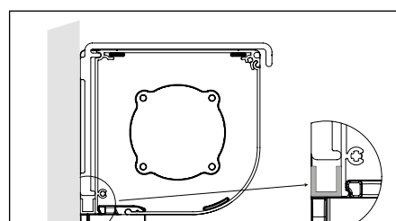
U-profil – horizontální
